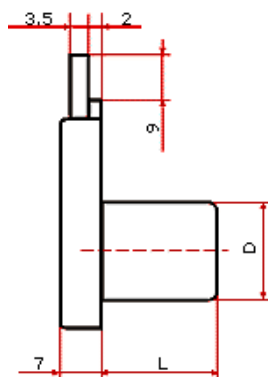
normální zámek
