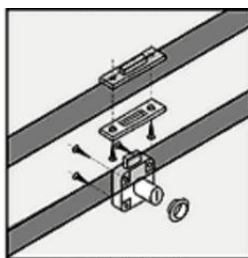
normální zámek
