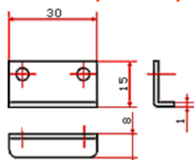
Protiplech PO6
