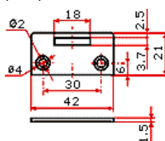
protiplech P07
