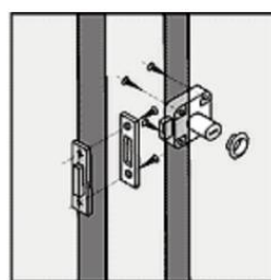
pravý zámek
